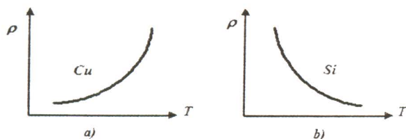
Figura C. Variación de la resistividad frente a la temperatura en: a) muestra de Cu, b) muestra de Si
